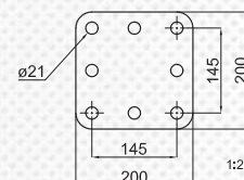
DIMENSIONI FLANGIA flange dimensions
