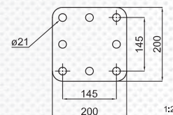
DIMENSIONI FLANGIA flange dimensions
